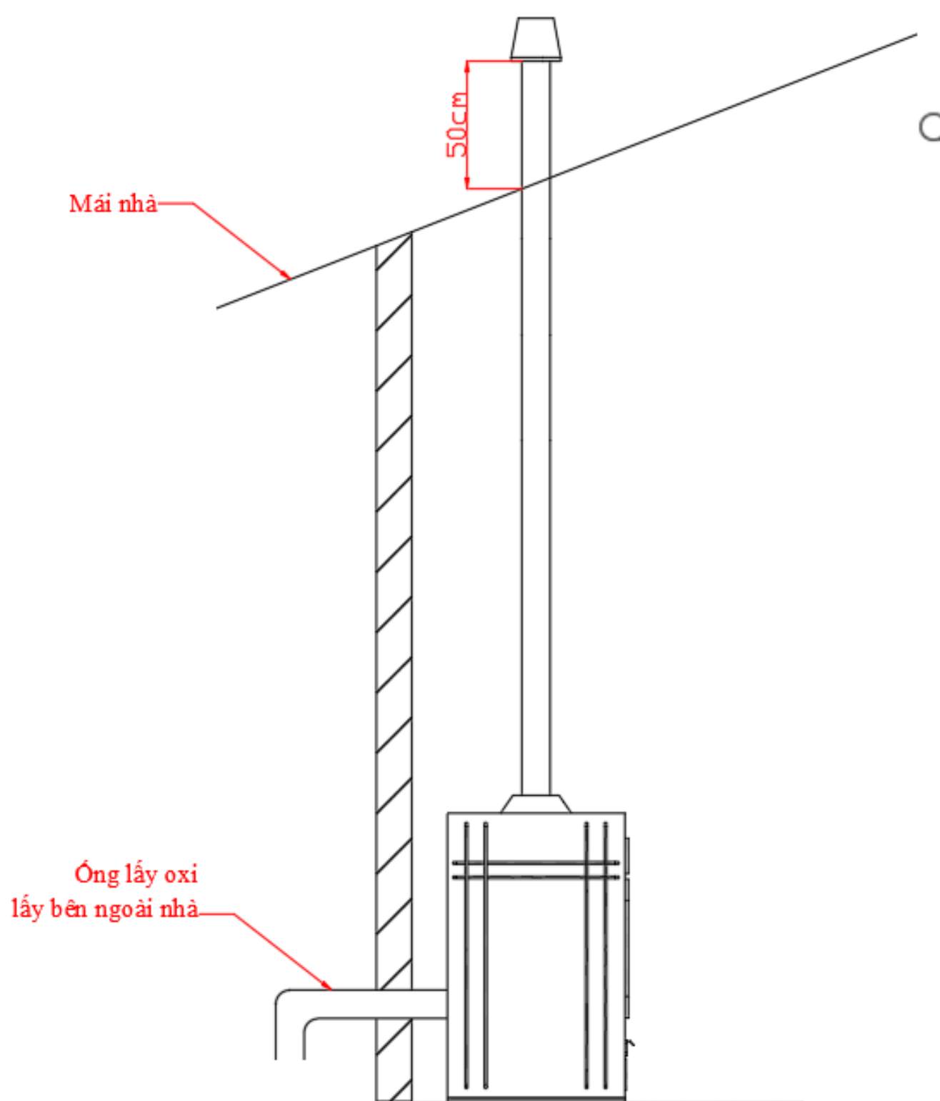
Sơ đồ lắp đặt ống khói chiều dọc
